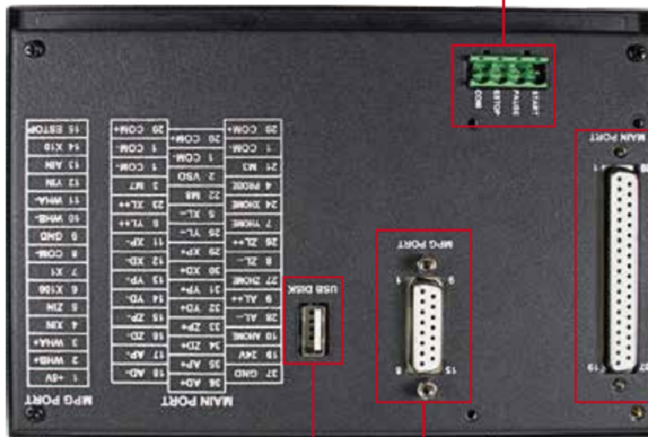
Start/Pause/Estop Switch
